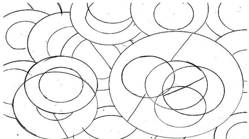
Hélice et rythme, Sonia Delaunay, 1937
